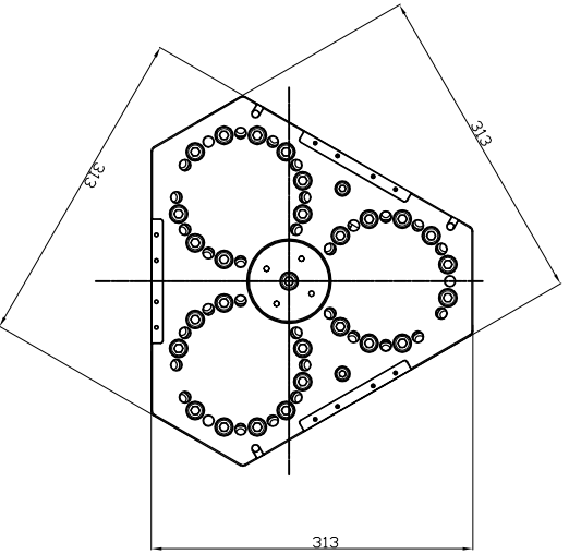
外形尺寸图 Dimensional outline drawing
