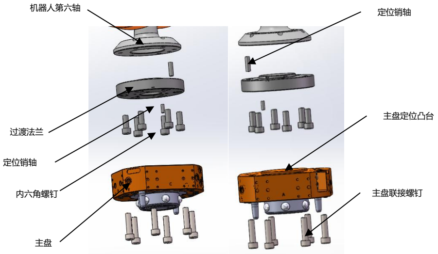
用过渡法兰联接主盘与机器人第六轴安装图
