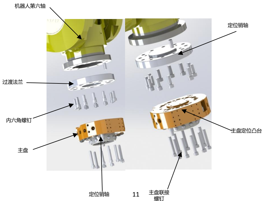
用过渡法兰联接主盘与机器人第六轴安装图
